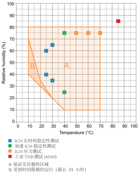
温湿度图表
